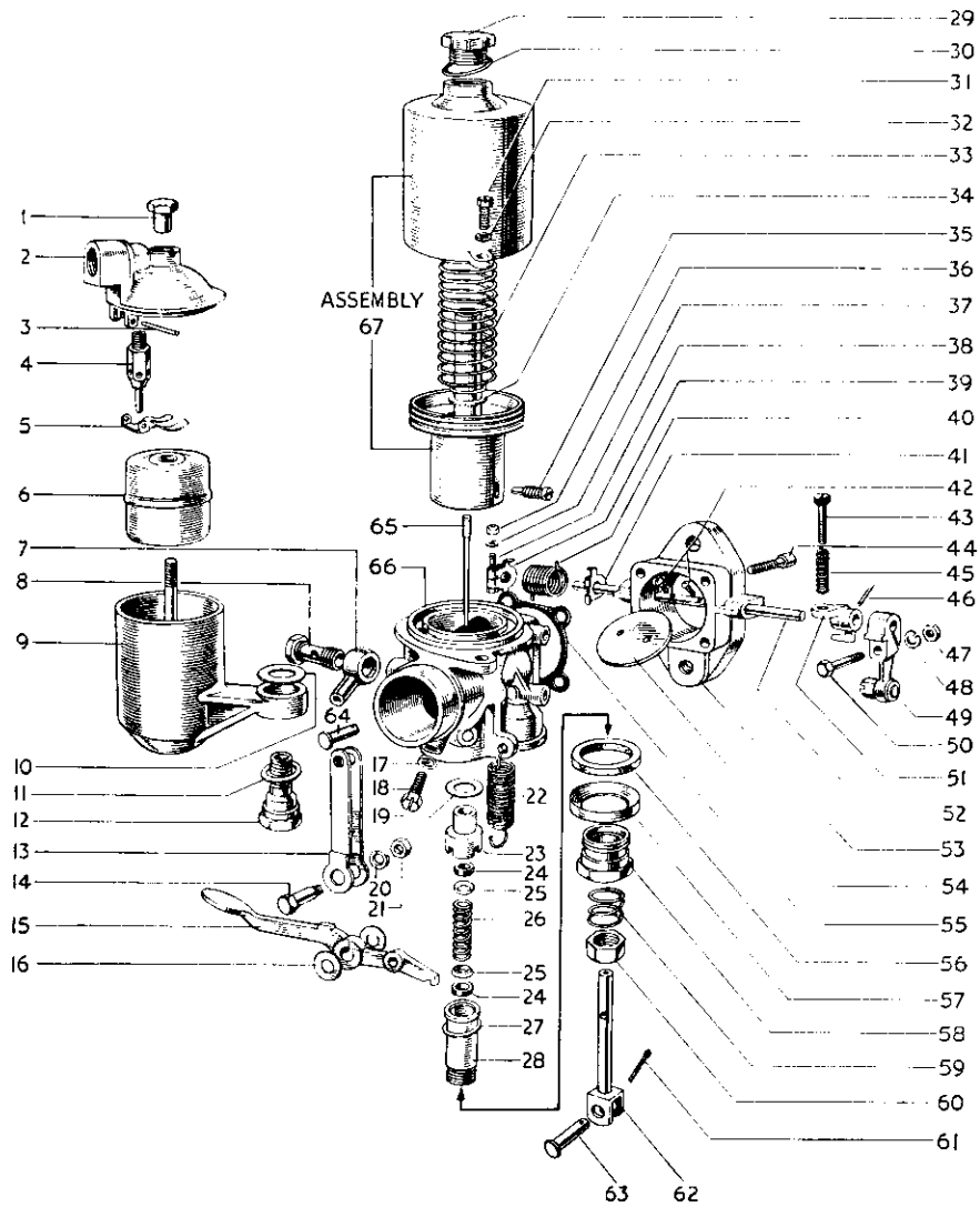
S.U. CARBURETTER
